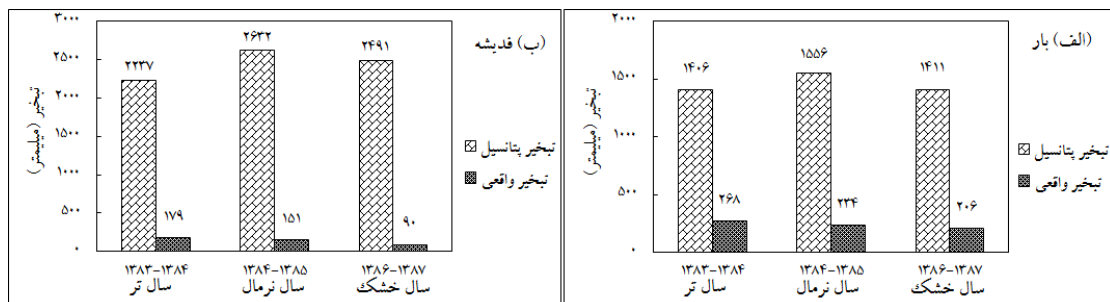
شکل ۷- مقایسه روند تبخیر- تعرق واقعی به دست آمده از الگوریتم سبال با تبخیر پتانسیل حاصل از تست تبخیر برای ایستگاه‌های (الف) بار و (ب) فدیشه
