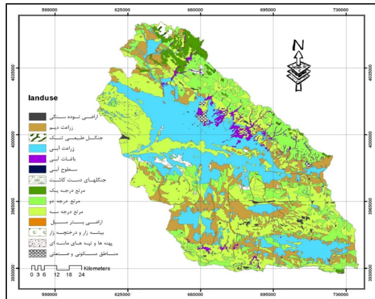
شکل ۵- نقشه کاربری اراضی حوضه آبریز نیشابور- رخ (شرکت آب منطقه‌ای خراسان رضوی، ۱۳۷۷)
