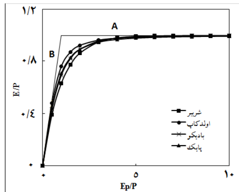
شکل ۲- نمایش چهار منحنی بادیکو (شربیر، اولدکاب، بادیکو و پایک)، خطوط مشخص شده با A و B به ترتیب شرایط با محدودیت آب و انرژی را نشان می‌دهد
