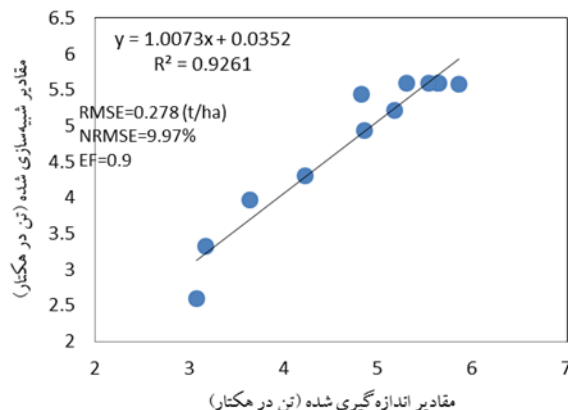
شکل ۴- نمودار مقایسه عملکردهای اندازه‌گیری شده و شبیه‌سازی شده
