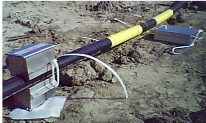
شکل ۳- دستگاه مغناطیس نصب شده بر روی لوله
