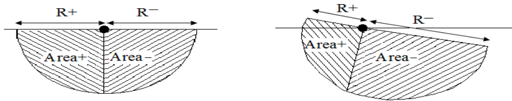
شکل ۱- پارامترهای مهم طراحی پیاز رطوبتی در اراضی شیب‌دار و مسطح
